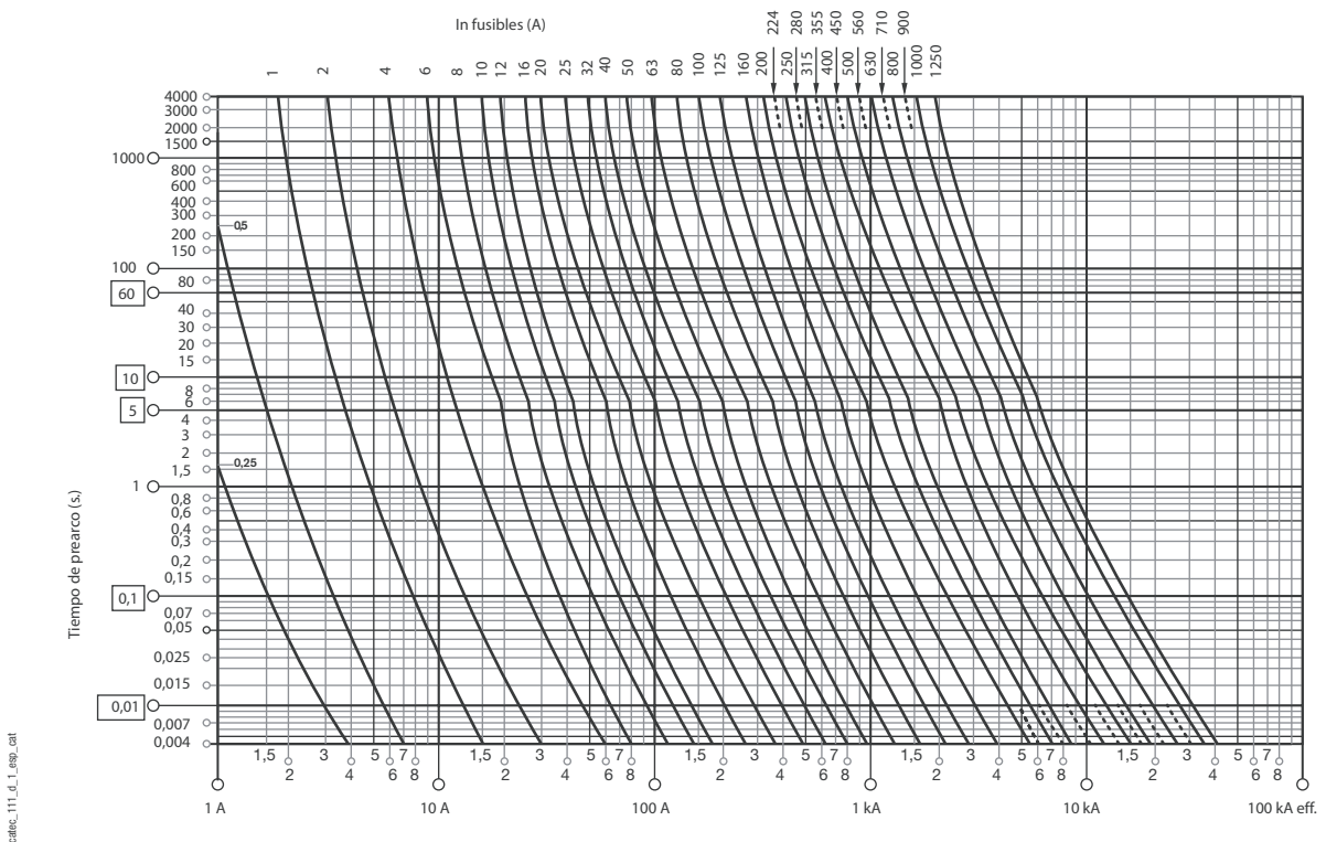
Características de funcionamiento tiempo/corriente
