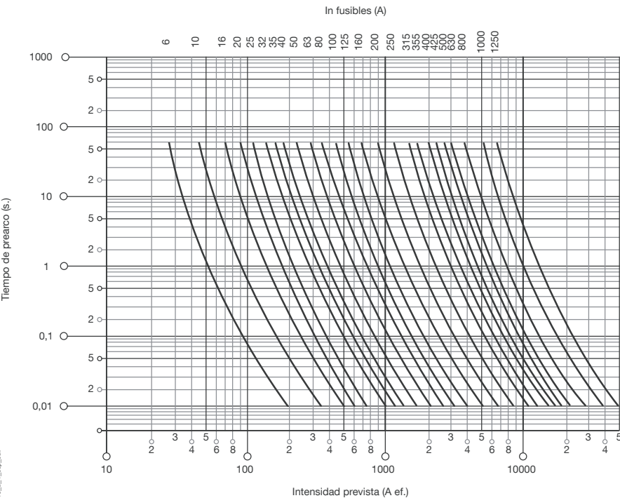
Características de funcionamiento tiempo/corriente
